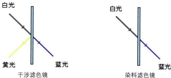
图1-2 滤色镜的滤色原理
