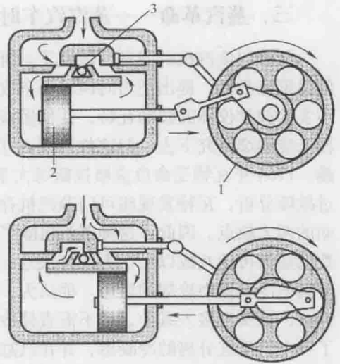
图1-1 瓦特蒸汽机
