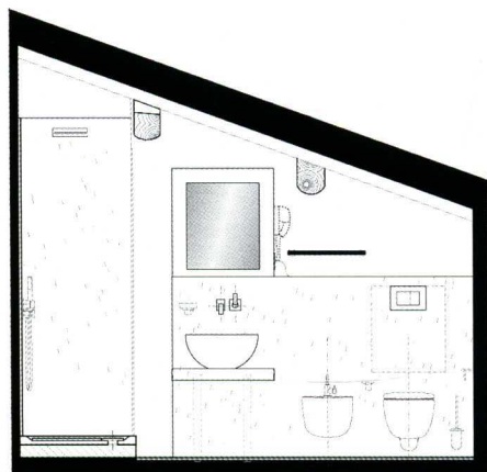
sezione sul bagno suite 5
