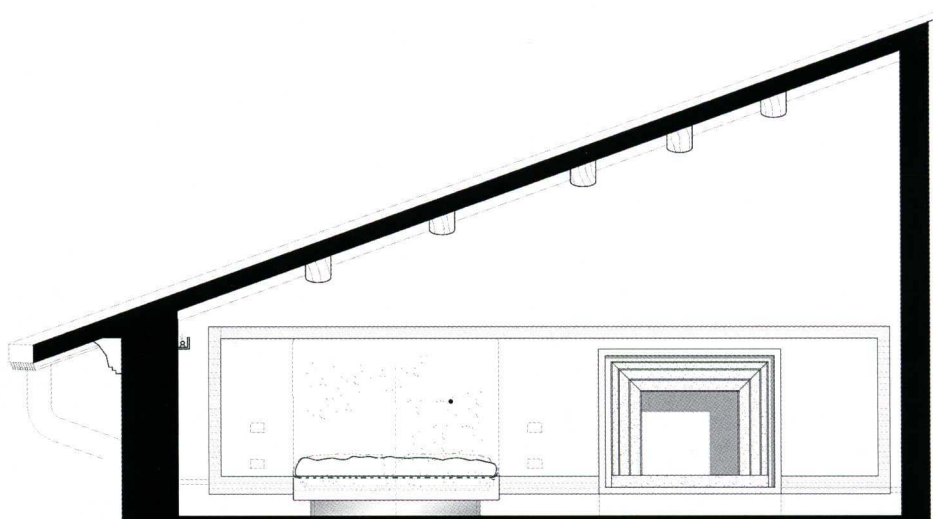
sezione sulla parete testata letto suite 5
