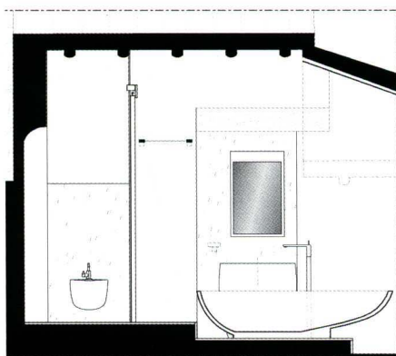
sezione sulla vasca suite 6
