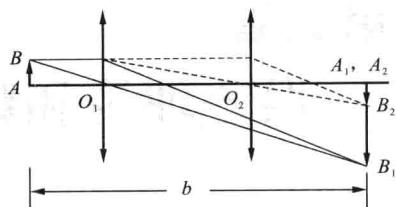
图 1-1-3 共轴调节
