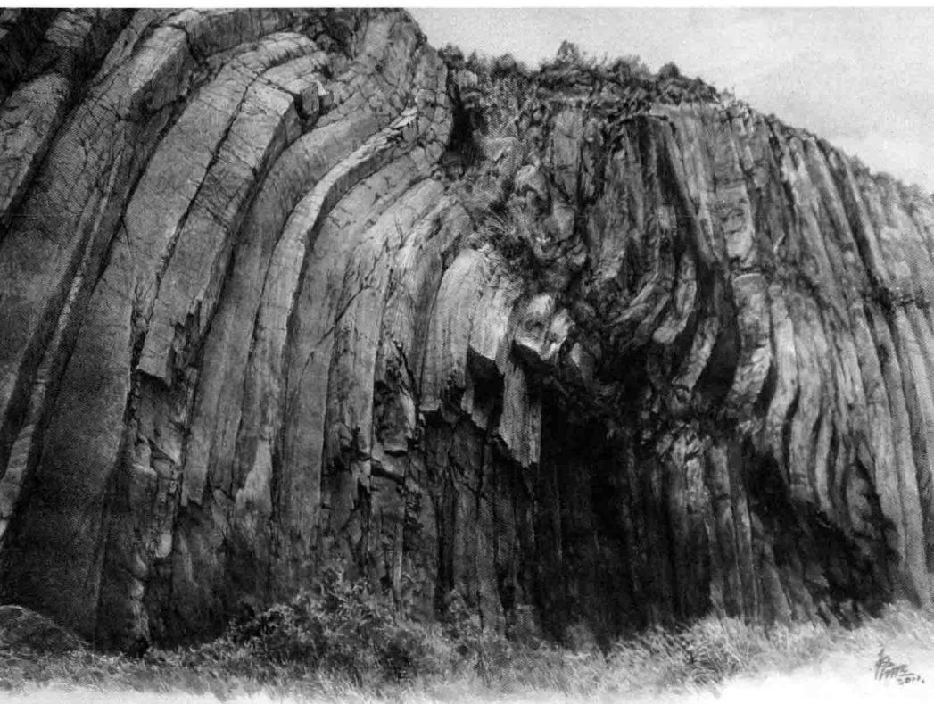
萬宜水庫流紋岩（2010）
