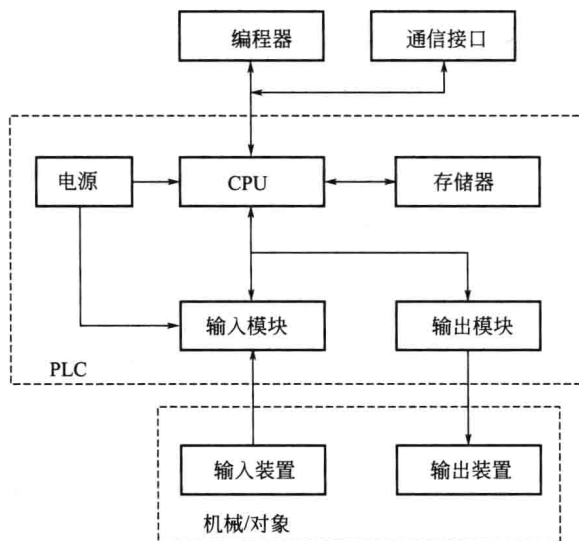
图 1-1 可编程控制器结构框图
