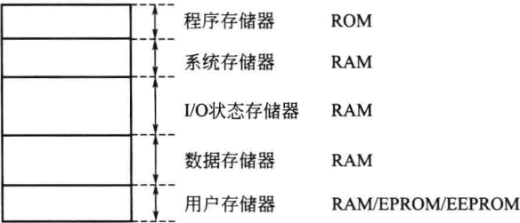
图 1-2 存储器的区域划分
