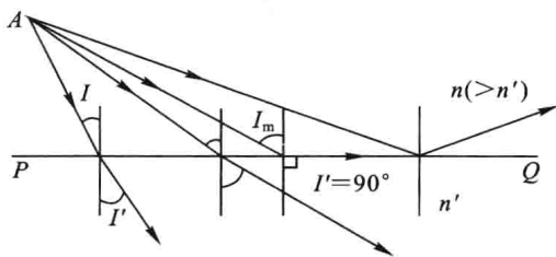
图 1-2 光的全反射现象
