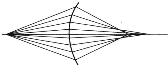
图 1-7 轴上点成像的不完善性
