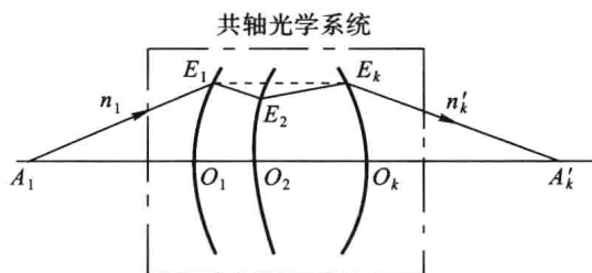
图 1-4 共轴光学系统及其完善成像
