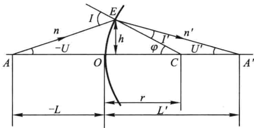
图 1-6 单个折射球面的折射
