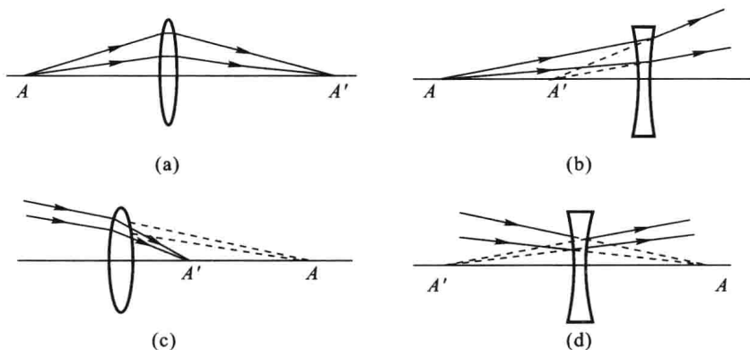
图 1-5 物、像的虚、实
