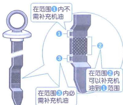
检查机油液面高度
