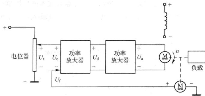
图 1-4 直流电动机转速闭环控制系统
