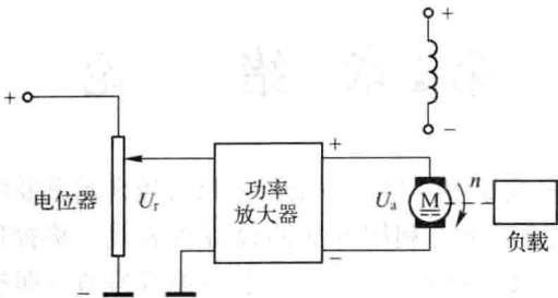
图 1-1 直流电动机转速开环控制系统原理图
