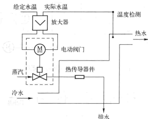
图 1-6 热力系统的闭环反馈控制
