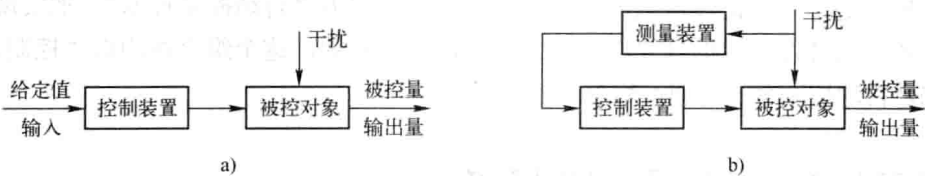
图 1-3 两种开环控制形式框图
