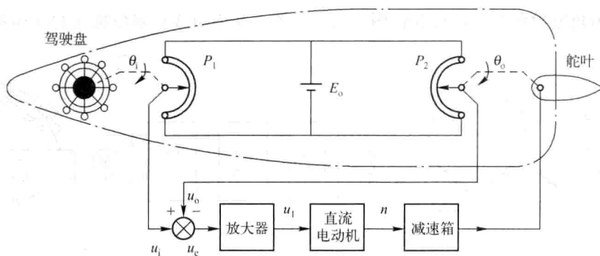
图 1-8 船舶随动舵的控制系统原理图
