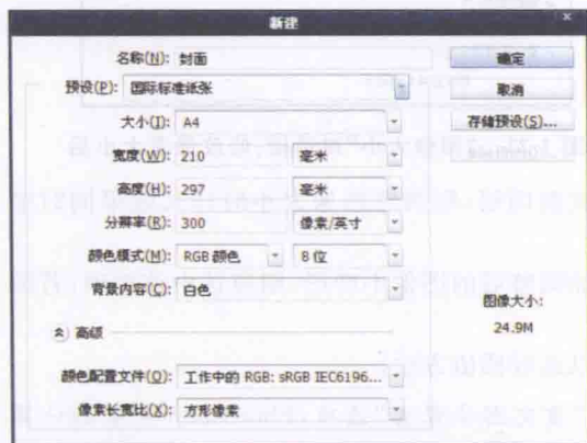
图 1-18 “新建”对话框
