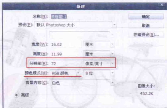
图 1-4 “新建”对话框
