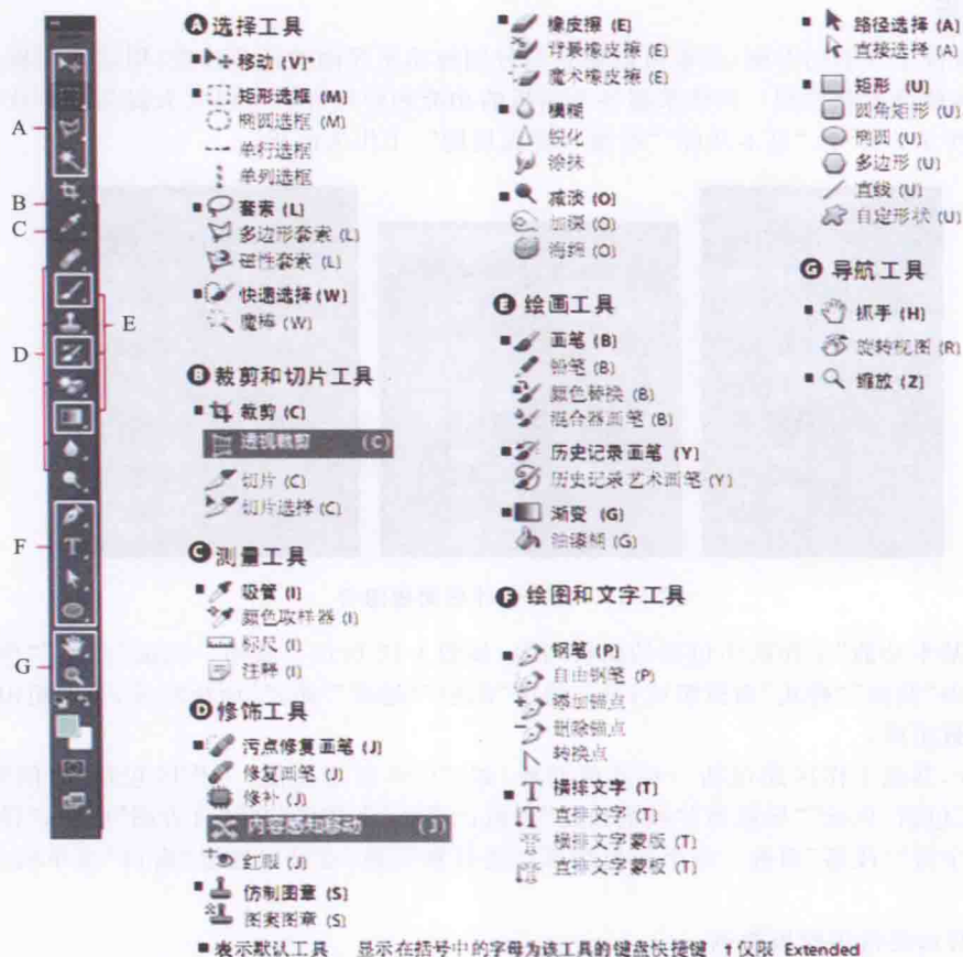
图 1-9 工具箱
