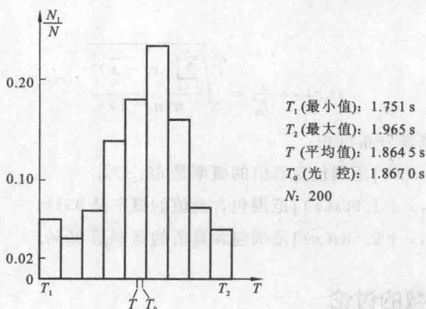
图 1.1 统计直方图
