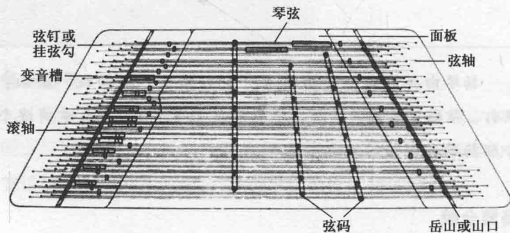
扬琴剖面
