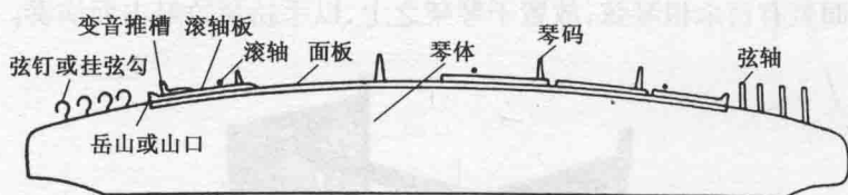
扬琴侧剖面
