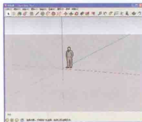
SketchUp 界面
