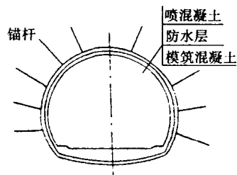
图 1.1.9 复合式衬砌
