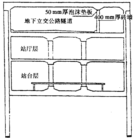
图 1.1.5 某地下铁道车站
