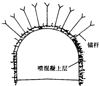
图 1.1.8 锚喷衬砌
