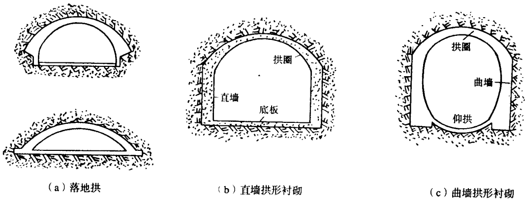
图 1.1.2 拱形衬砌
