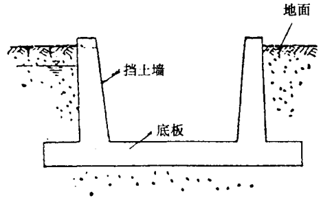
图 1.1.7 开敞式结构
