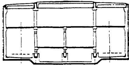
图 1.1.12 装配式密肋板车站
