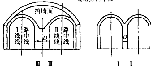
图 1.1.4 连拱形衬砌
