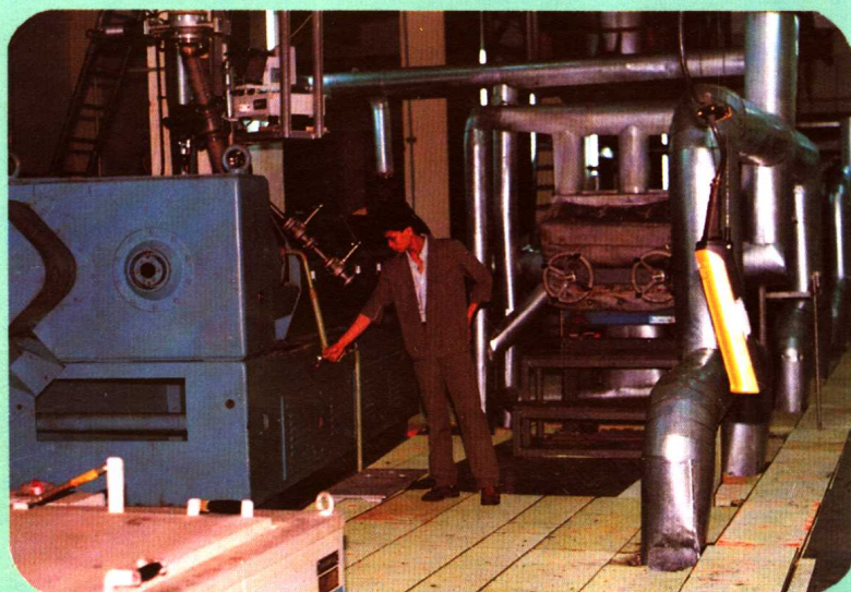
前纺车间引进的蜗杆挤压机
