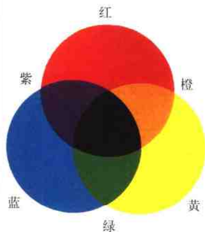
▲ 原色与间色
