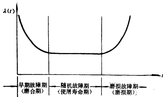
图1-2 故障率曲线(浴盆曲线)
