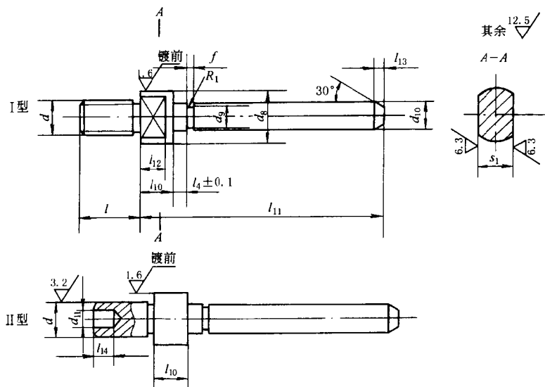
B 型手柄杆
