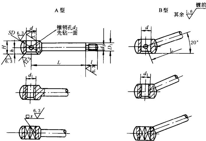
球头手柄（JB/T 7270.8—1994）
