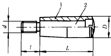
1—转套；2—螺钉
