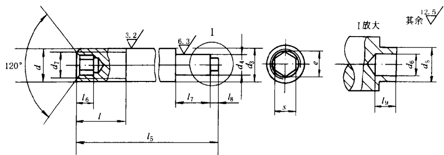
A 型手柄杆
