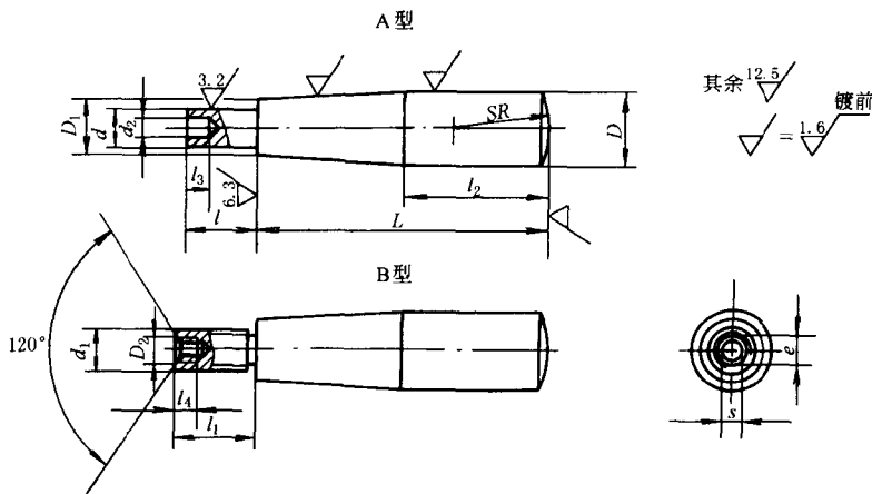
手柄 (JB/T 7270.1—1994)
