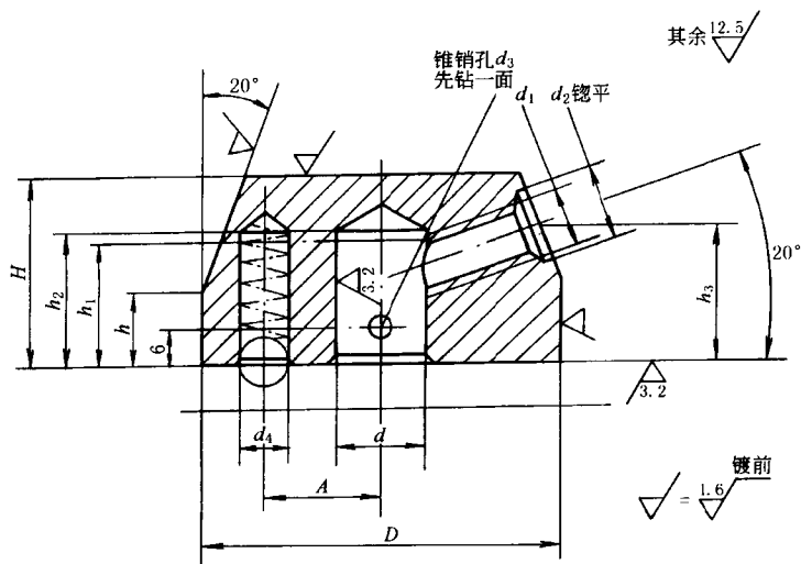
定位手柄座 (JB/T 7272.4—1994)
