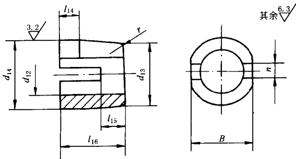
弹 性 套
