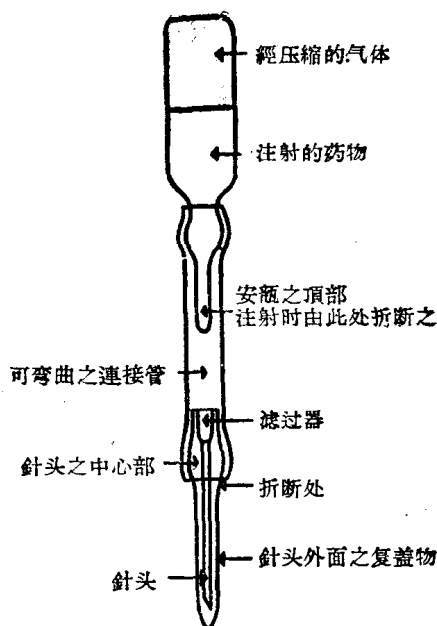
图1 自动注射器
