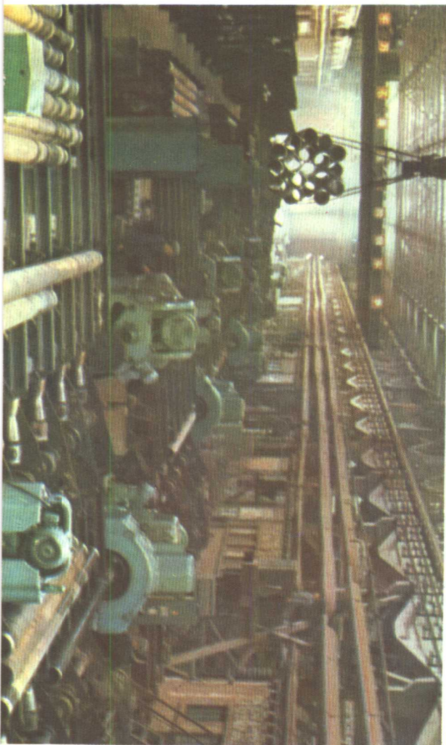
③ 无缝钢管厂 Seamless Steel Pipe Plant 新疆维吾尔自治区 乌鲁木齐市
