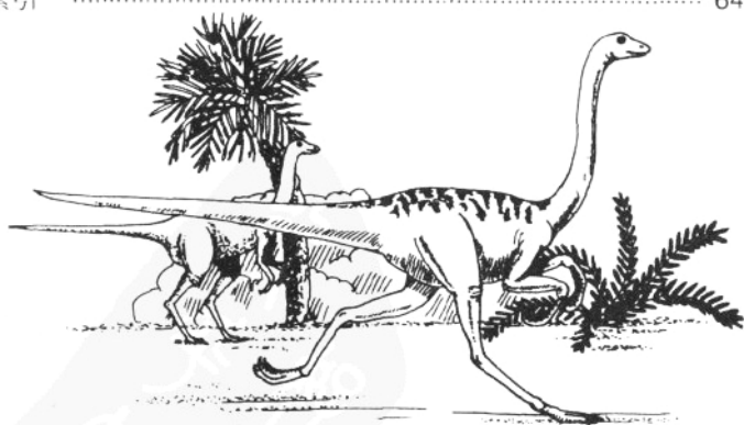
Ornithomimus (似鸟龙)
