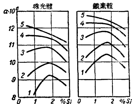
圖4 矽對生鐵綫膨脹係數的影響：
