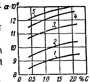
圖9 銅對生鐵綫膨脹係數的影響：
