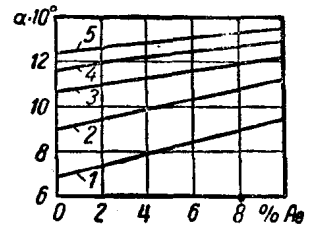
圖8 鋁對生鐵綫膨脹係數的影響：
