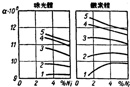
圖5 鎳對生鐵綫膨脹係數的影響：
