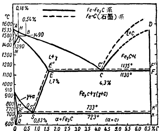
圖 1 鐵—碳平衡圖。
