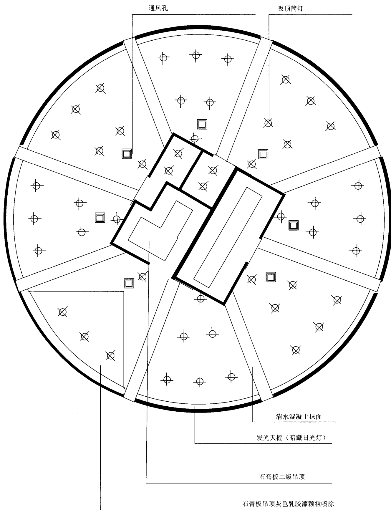
美容美发中心天花布置图(详见彩页第4页)
