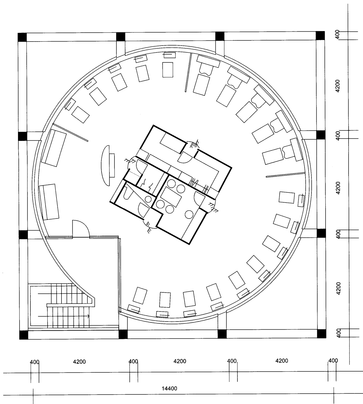
美容美发中心平面布置图 (详见彩页第4页)
