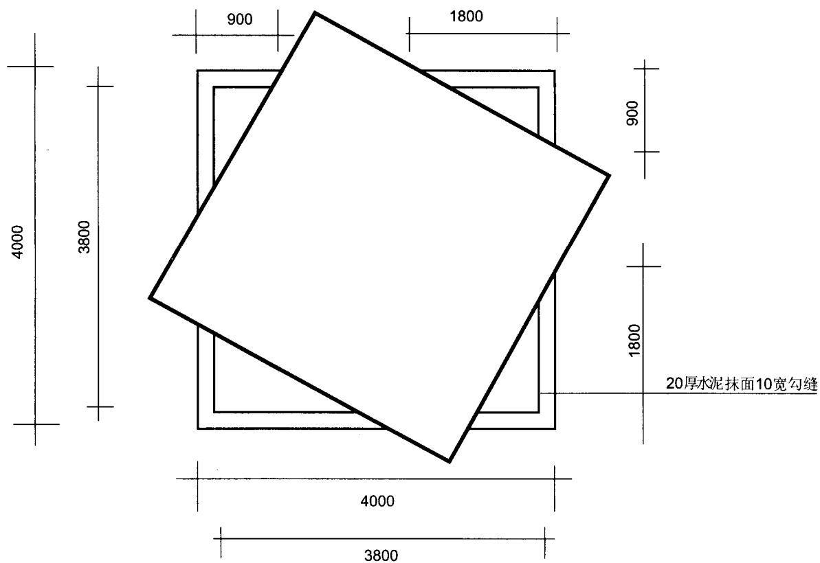
中心办公区地面大样
