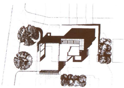
总平面图
