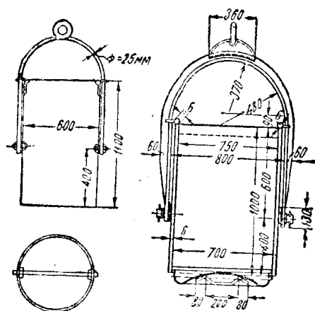
圖2 圓形翻倒式金屬吊斗
