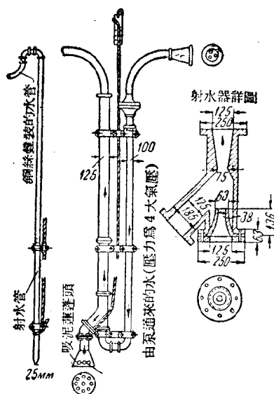
圖 5 水力吸泥機
