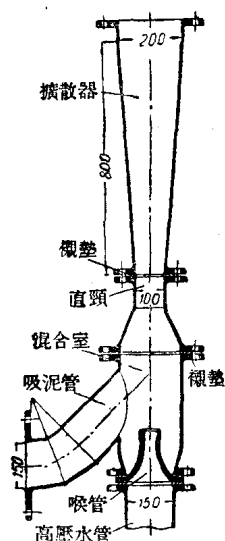
圖 7 裝有列奧諾維奇式射水器的水力吸泥機
