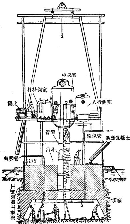
圖 10 在沉箱基礎上建造基礎的工作圖
