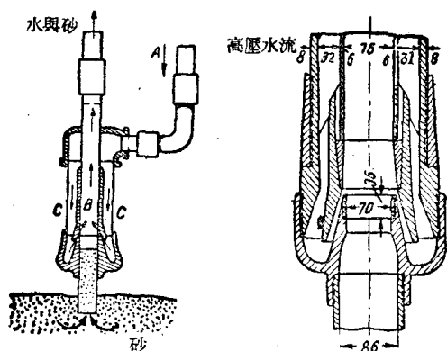
圖 6 水力吸泥機（作用圖及詳圖）
