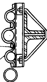
40×40×4 角钢支架 钢管沿钢屋架敷设
