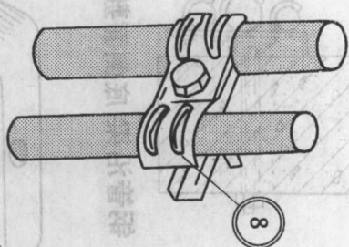
管卡使用三式
