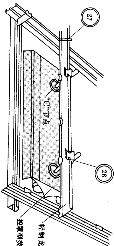
荧光灯具在轻钢龙骨上做安装示意图之一
