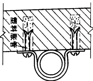
钢管沿墙敷设
