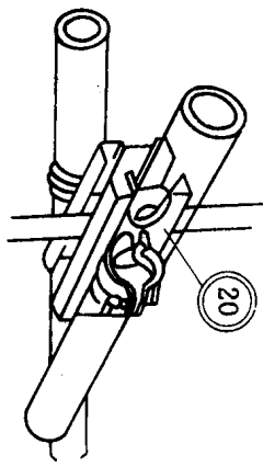
圆钢夹板管卡安装示意图
