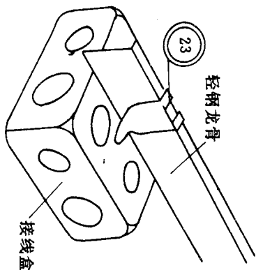
接线盒固定在方形 轻钢龙骨上安装示意图
