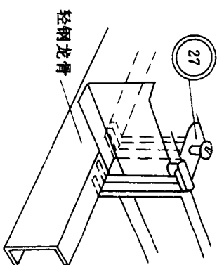
龙骨连接卡安装示意图
