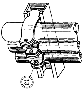
夹板式管卡垂直安装示意图
