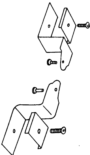
24 连接龙骨固定卡组装图 (定货编号: HXS341)
