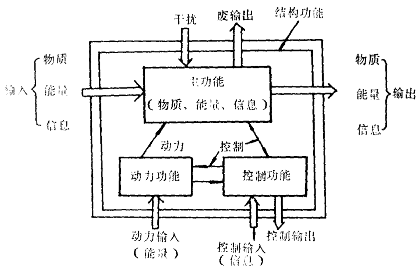
图 1-3 机电一体化系统的功能构成
