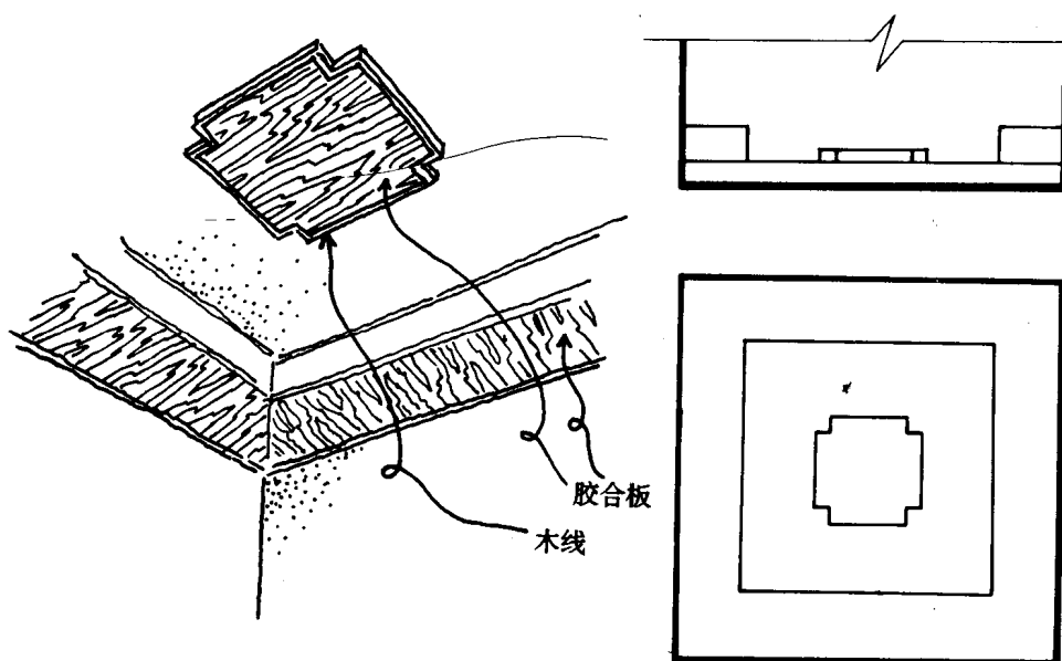
图 3 灯心板的设计及施工示意图
