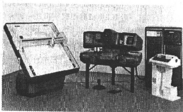
图 1-3-5 AC1 解析立体测图仪
