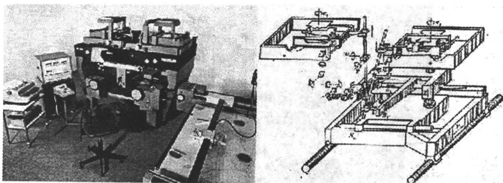
图 1-2-5 A10 立体测图仪
