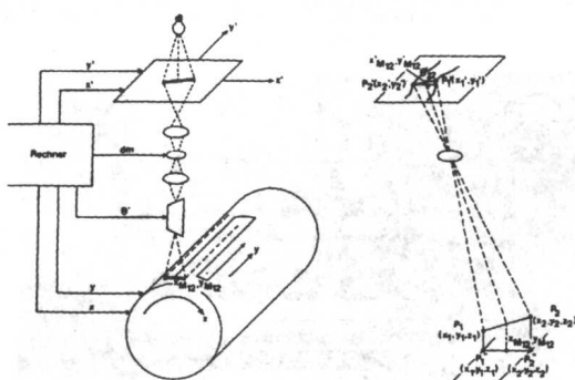
图 1-3-7 正射投影仪 OR1 及其原理图
