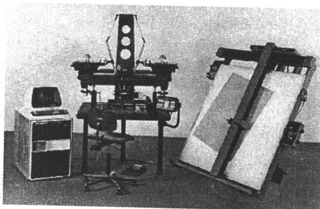
图 1-2-7 AG1 立体测图仪
