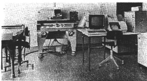
图 1-3-2 AP/C3 解析立体测图仪
