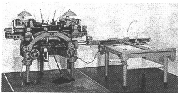
图 1-2-3 Stereoplanigraph B 立体测图仪(光学-机械投影)
