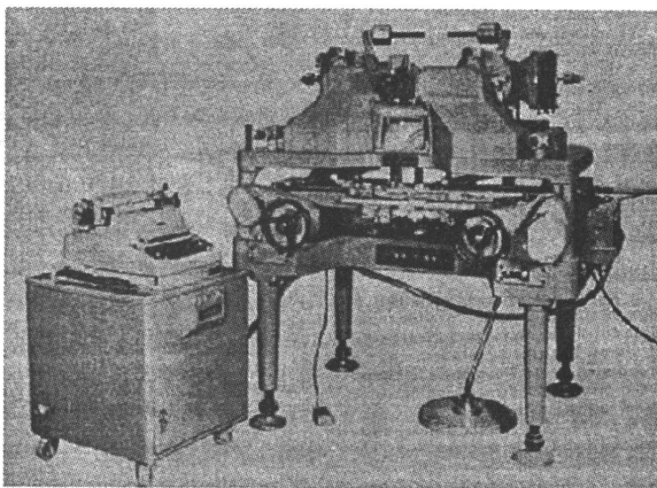
图 1-2-3 Stereoplanigraph B 立体测图仪(光学-机械投影)
