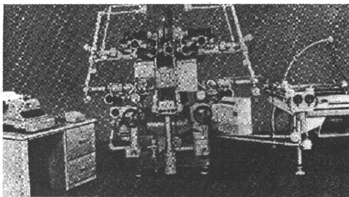
图 1-2-2 Stereoplanigraph C8 立体测图仪(光学投影)
