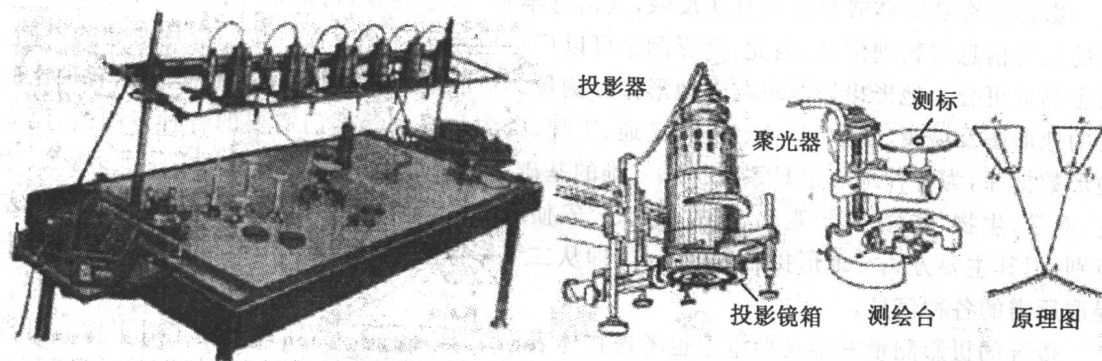
图 1-2-1 多像仪(光学投影)
