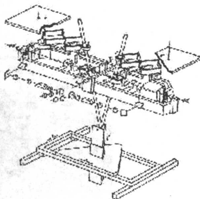
图 1-2-4 A8 Autograph 立体测图仪(机械投影)
