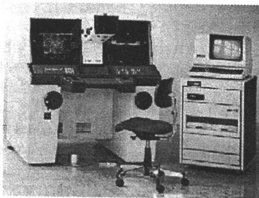
图 1-3-4 DSR11 解析立体测图仪
