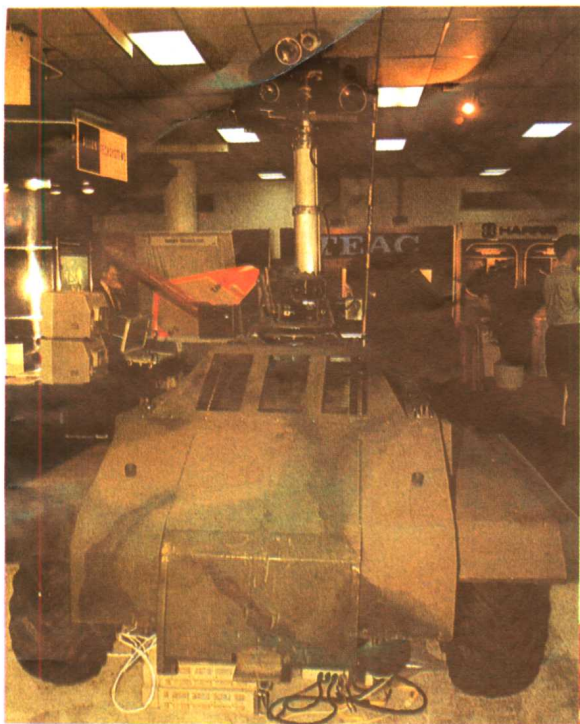
远程遥控侦察车,由加拿大研制,总重量 10.4 公斤,最大时速 5 公里,车顶部设有自动升降的潜望镜,它具有侦察、监视、传声等多种功能。
