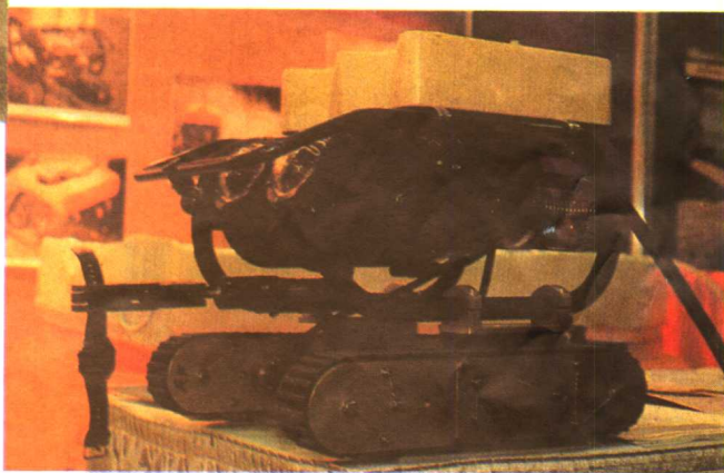
特警部队的深海调查测用车,该车能在警员的遥控下到 50M 深的海底搜索目标。
