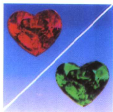
Alexandrite 变石
