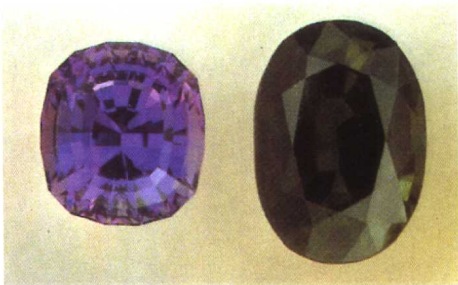
Corundum 刚玉
