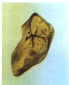
Amber 琥珀
