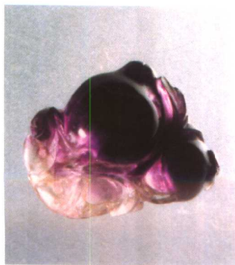
Amethyst 紫晶
