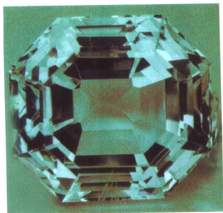
Apophyllite 鱼眼石
