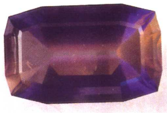
Cordierite
