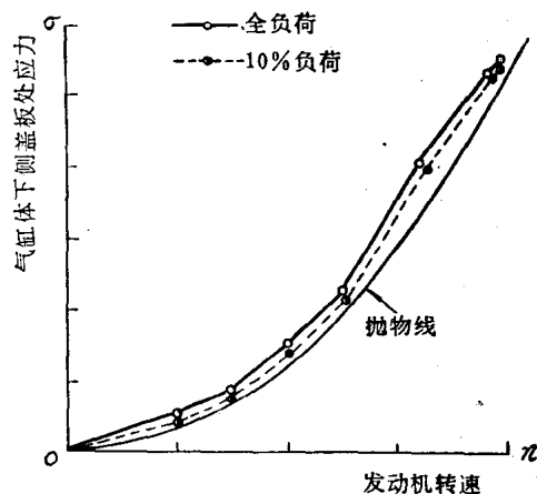
图4-1-1 发动机转速、负荷及缸体应力的关系
