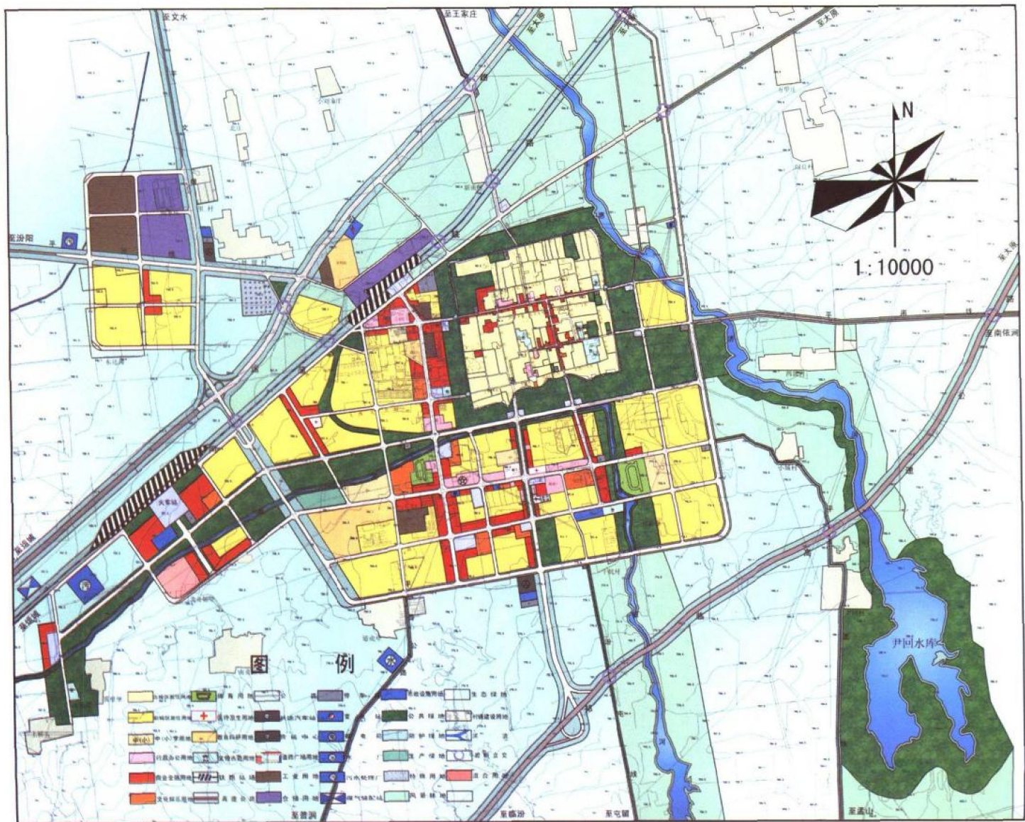
图6 总图
