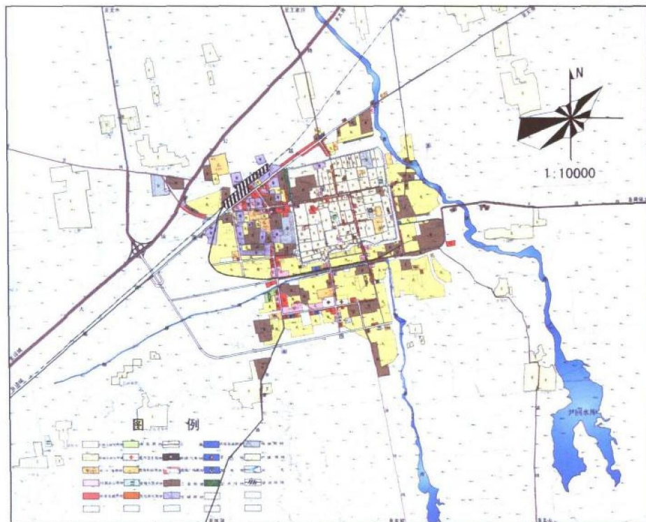
图5 现状图
