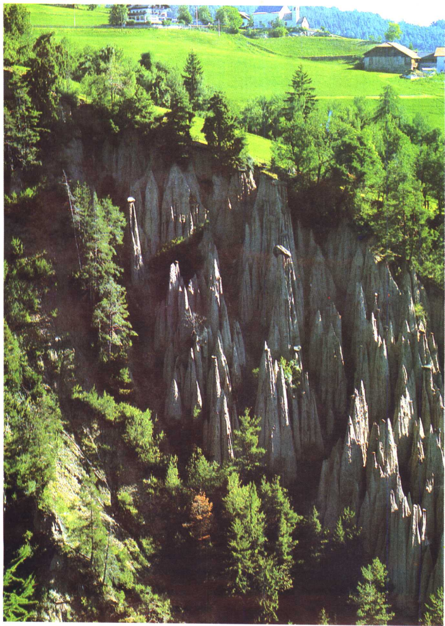
意大利里农奇异的土金字塔，是冰川冰碛物的残迹
