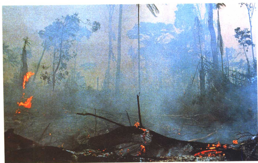
森林大火释放出二氧化碳
