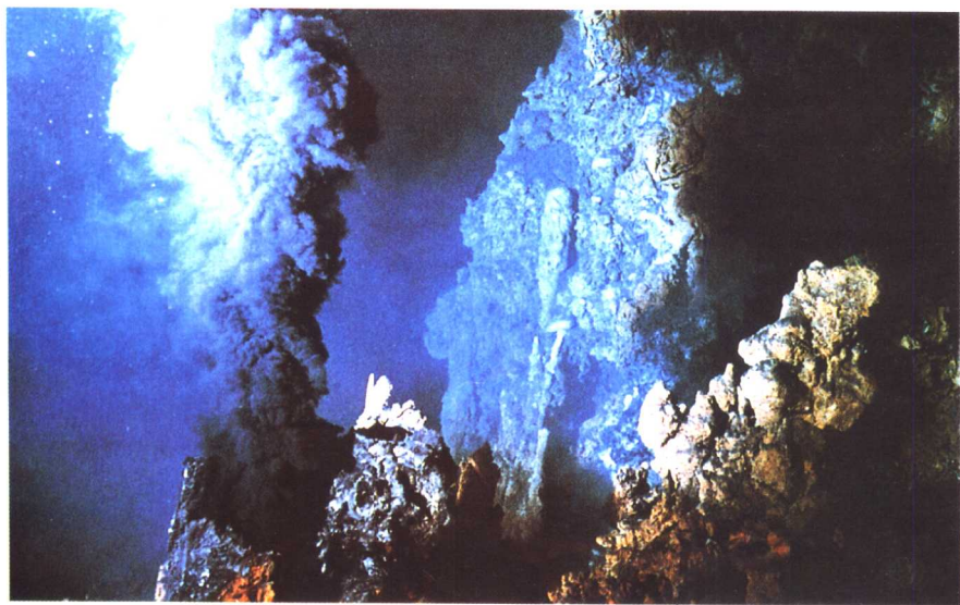
1979年在东太平洋海岭发现的黑烟筒
