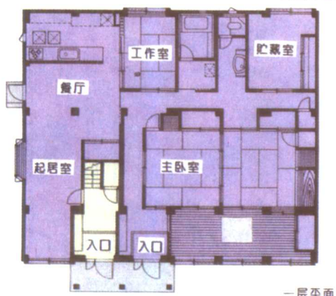
一层平面
