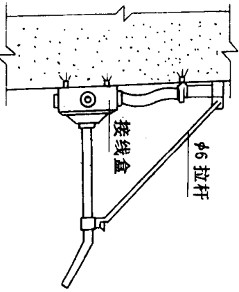
灯具在柱上安装
