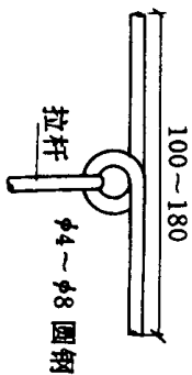
灯具在钢屋架上安装
