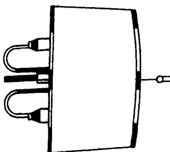
HD2024-2 3×40 瓦 φ400×360 3.5 千克
