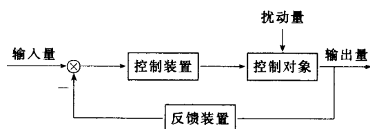
图 1-5 闭环控制系统方框图
