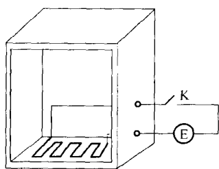
图 1-2 炉温开环控制系统
