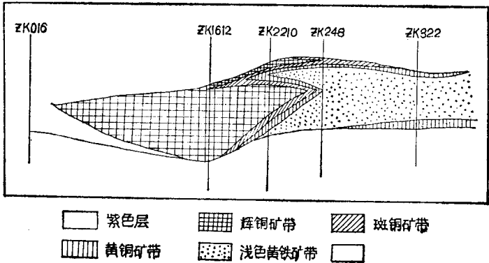
图 8 云南六苴矿区矿物分带示意图
