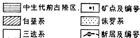
图 1 滇中砂岩铜矿分布示意图
