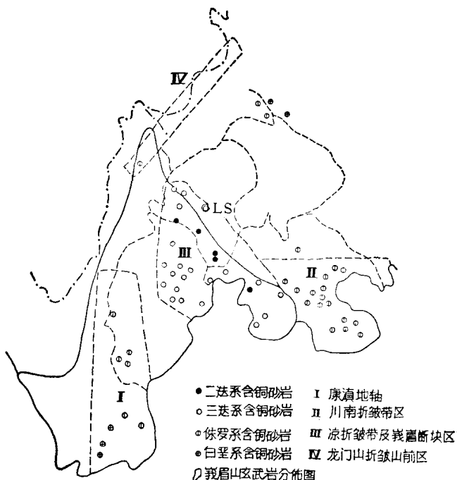
图4 四川砂岩铜矿分布示意图
