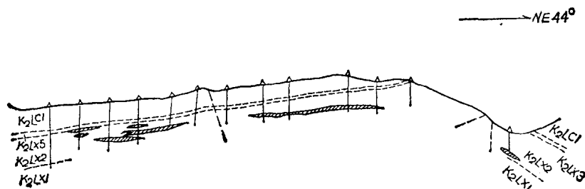
图5 云南郝家河矿床40号剖面图
