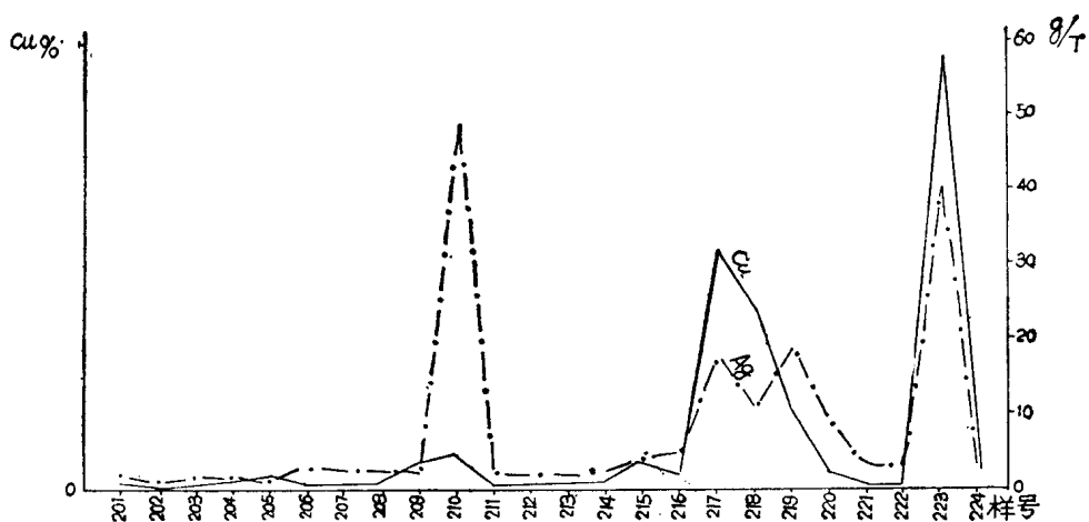
图 11 湖南九曲弯铜矿区 Cu、Ag 含量曲线图
