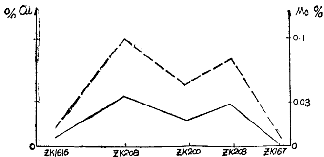
图 12 云南格依纳 Cu、Mo 含量曲线
