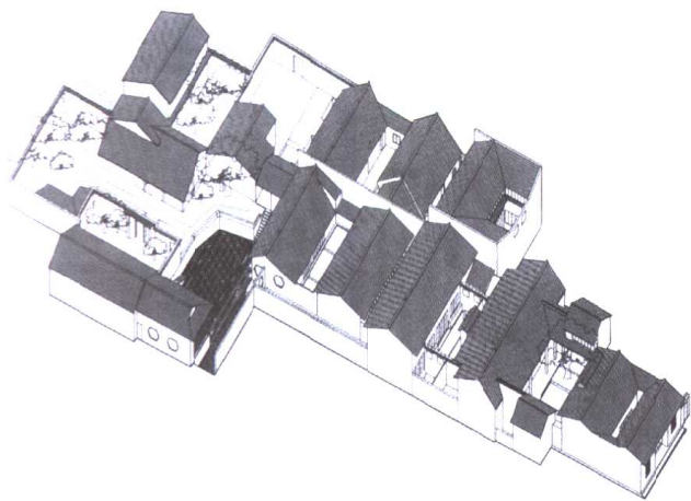
周庄张厅轴测图
