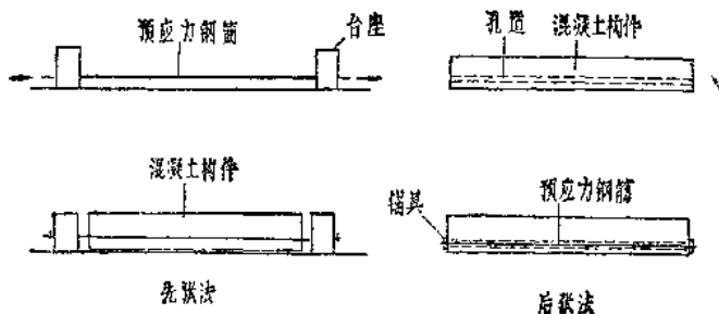
图 1-2 先张法与后张法
