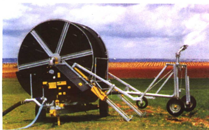
移动式卷盘 喷灌机
