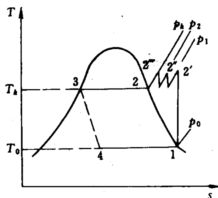
图 1-9 多级蒸汽压缩式制冷循环
