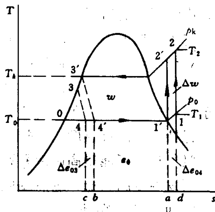
图 1-7 液体过冷和吸气过热循环
