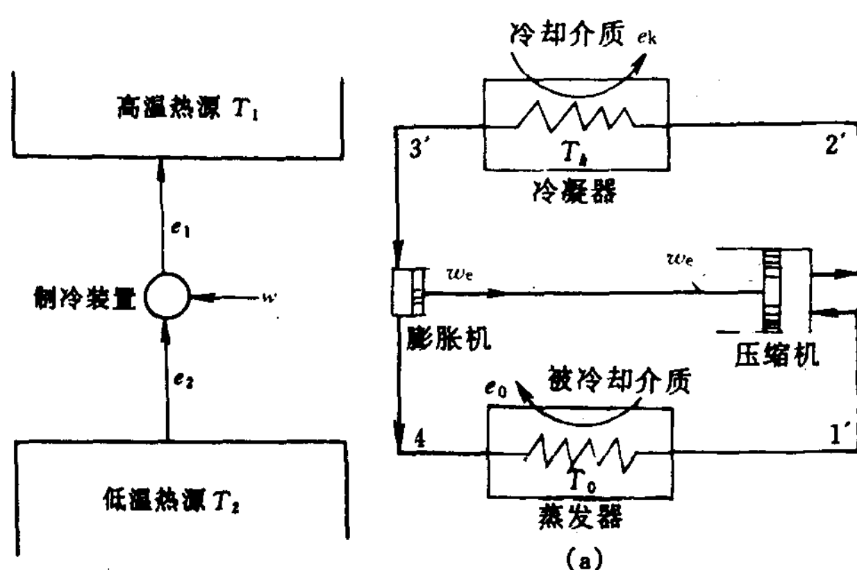
图 1-2 制冷装置与外界的关系
