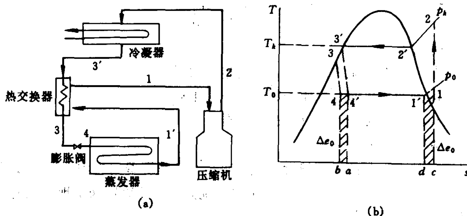
图 1-8 回热制冷循环及其 T-s 图
