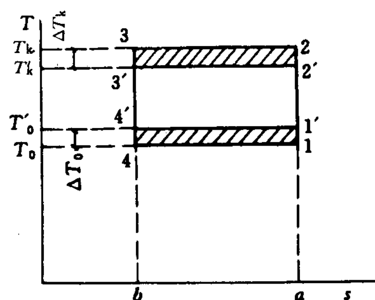
图 1-4 具有传热温差的逆卡诺循环
