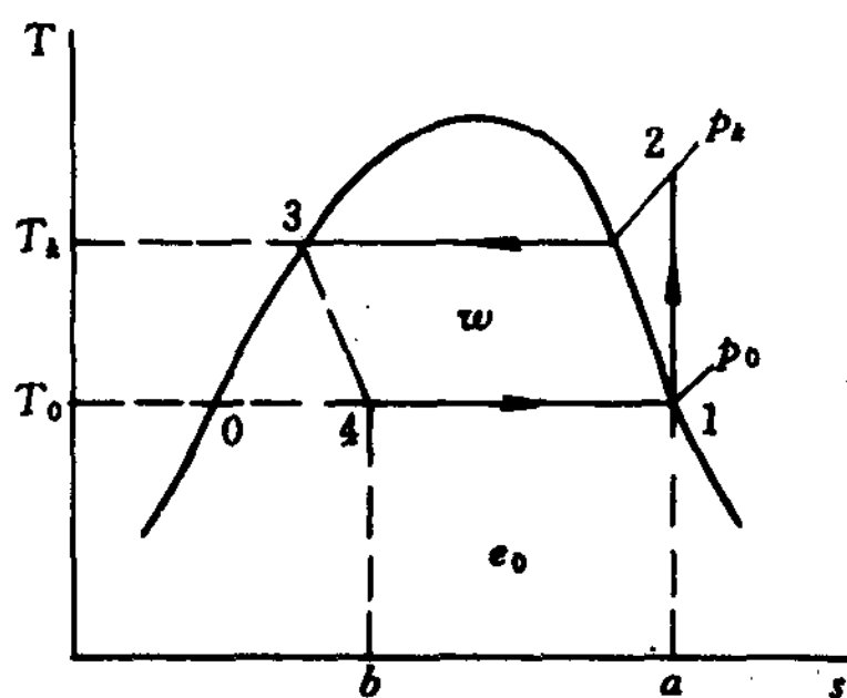
图 1-5 理论制冷循环的 T-s 图
