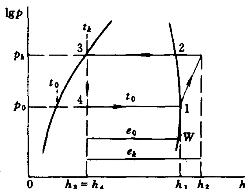
图 1-11 蒸汽压缩制冷理论循环的 \lg p-h 图
