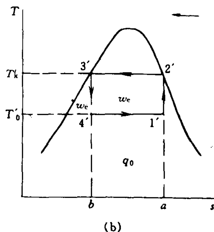
图 1-3 逆卡诺循环过程
