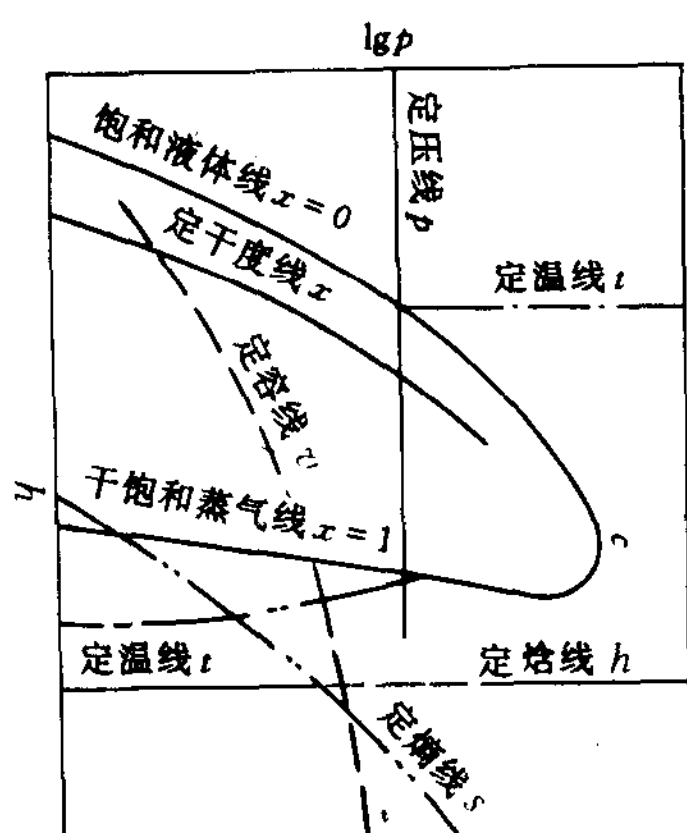
图 1-10 制冷剂的 \lg p-h 图
