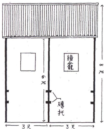
正面图
