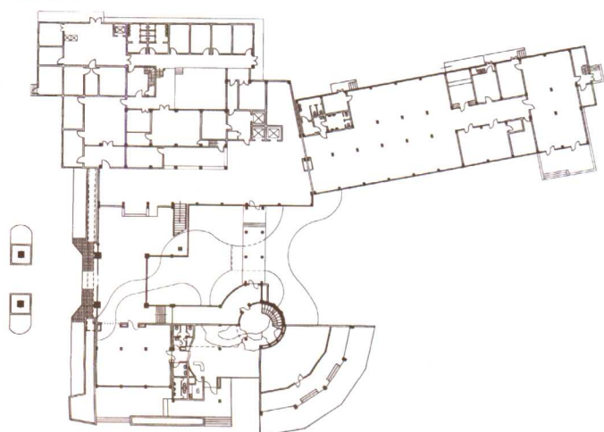
底层平面
