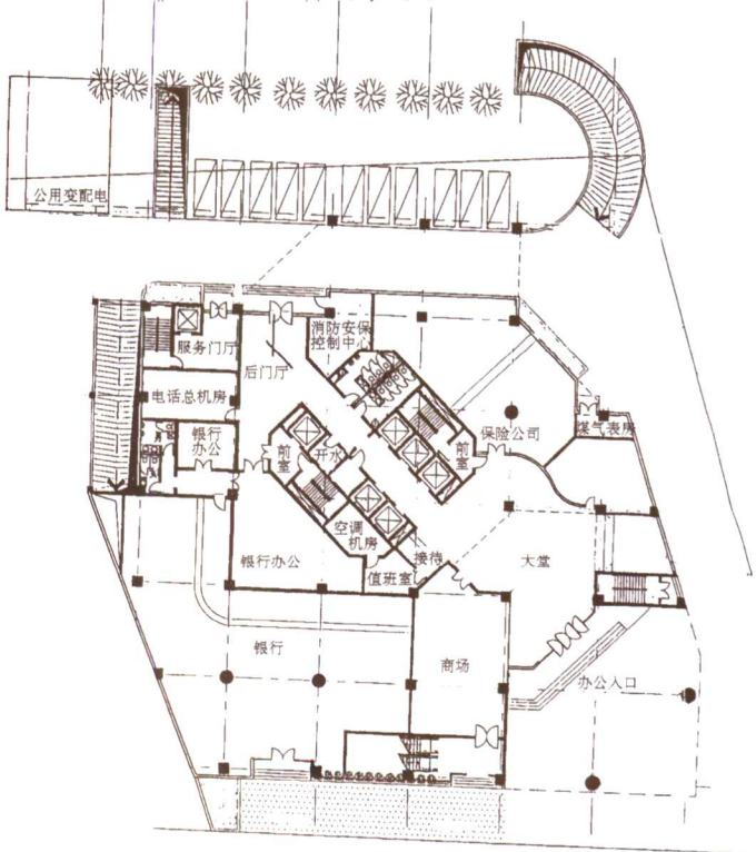
底层平面
