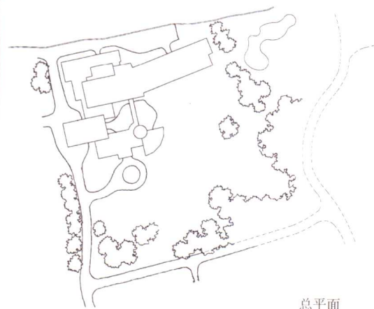
总平面
