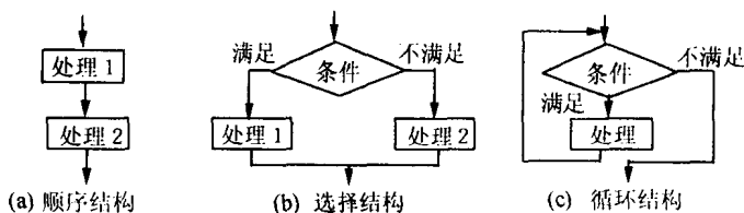
图 1.7 传统结构化流程图的基本图
