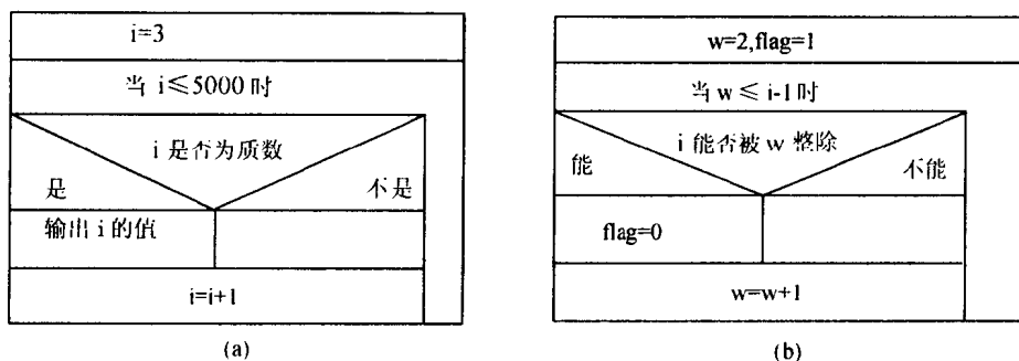
图 1.11 输出 3~5000 之间所有的质数
