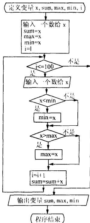
图 1.6 传统流程图的应用
