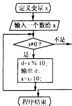
图 1.5 用传统流程图表示算法
