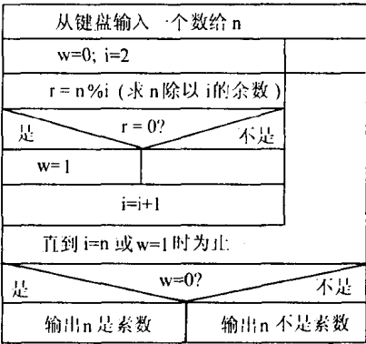
图 1.10 判断素数的 N-S 流程图
