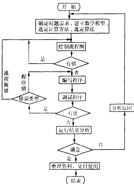
图 1.8 程序设计的工作流程
