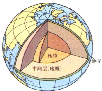
地球的内部构造
