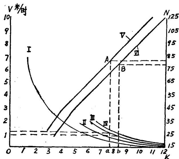
图 1-3 摆球硬度与岩石可钻性关系
