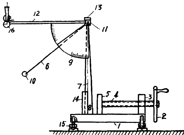
图 1-2 摆球硬度仪
