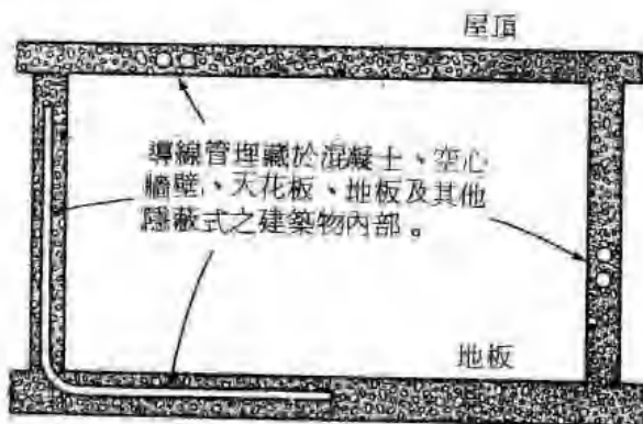
圖 7—5 暗管配裝
