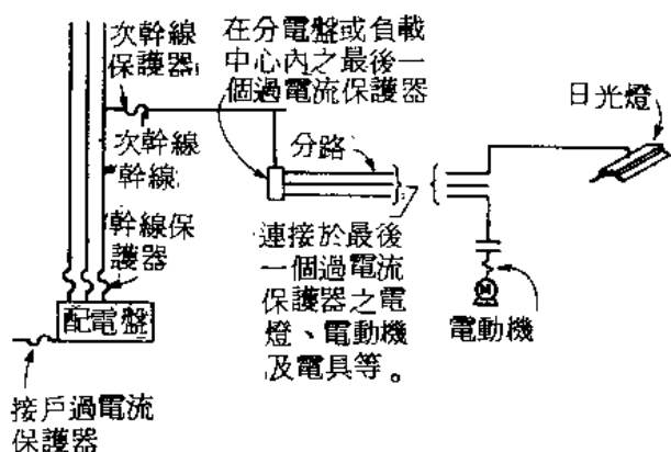
圖 7-1 分路之定義
