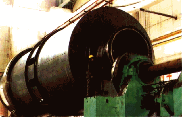
▶ 唐山冶金矿山机械厂为秦皇岛港粮食码头生产的高强度胶带输送机
