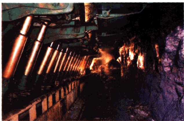
▲开滦综机采煤工作面
