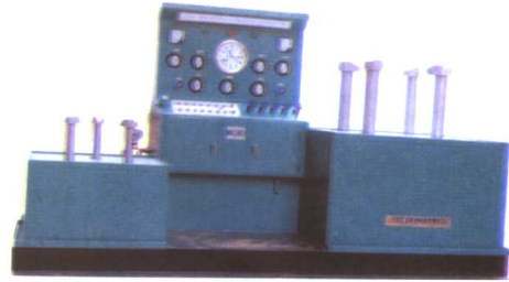
YFC-D型液压蝶阀测试机
